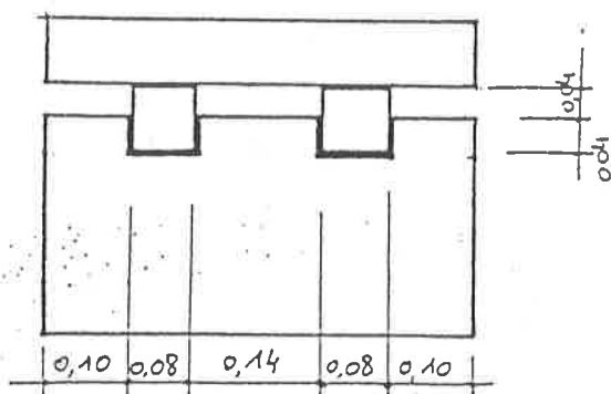
ZIJAANZICHT
